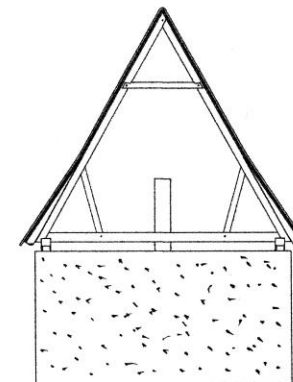
pohled Severní
