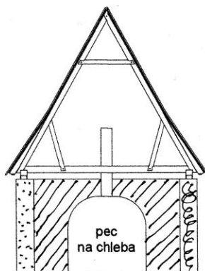
pohled Jižní
